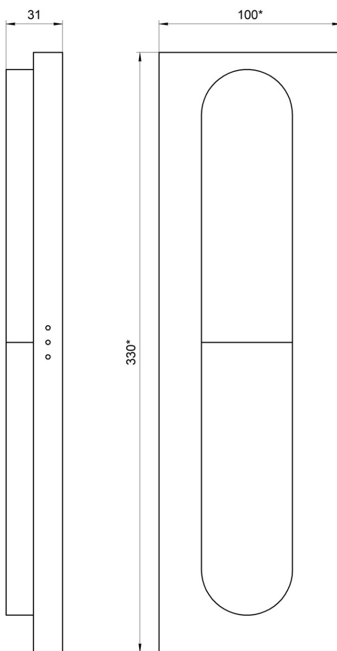
Рис.1 Внешний вид «Указатель лифтовой» НШЕК.468232.204
